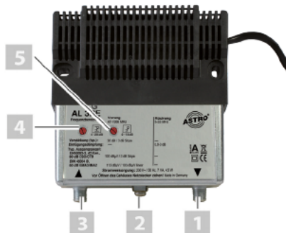
Bild 1: AL 3RE
