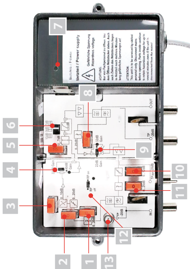
Bild 2: Verstärker HVO V40 P, Innenansicht
