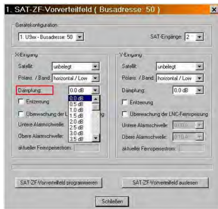
Bild 5: SAT-ZF-Vorverteildfeld, Dämpfung einstellen
