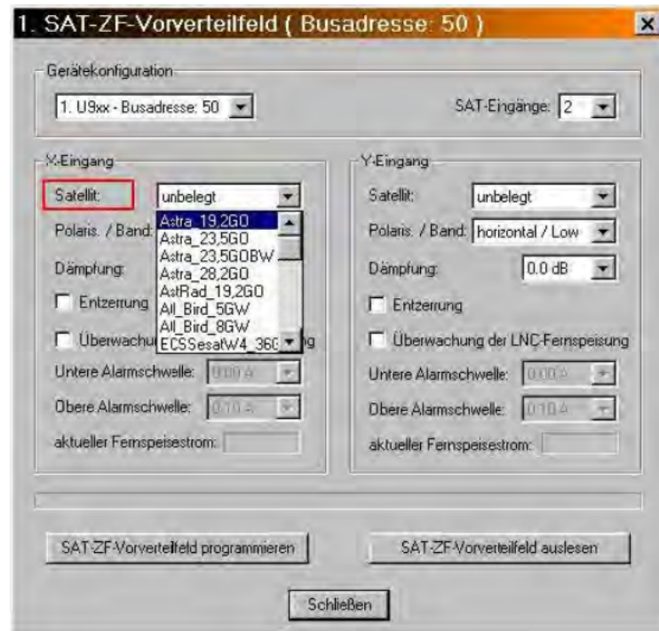
Bild 4: SAT-ZF-Vorverteildfeld, Eingänge belegen
