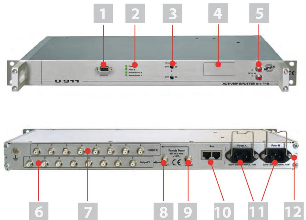
Bild 1: U 911 SAT-Verteilerfeld
