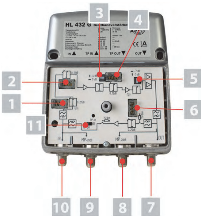
Bild 2: Verstärker HL 432 G, Innenansicht (HL 433 G identisch)
