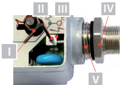
Bild 3: Eingangs- und Ausgangsbuchse montieren
