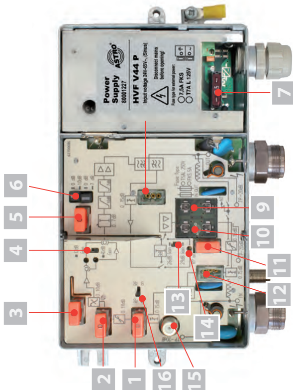
Bild 2: Verstärker HVF V44 P-PG11, bestückt mit 2 x 3,5/12“ Buchsen und 2 x F-Buchse
