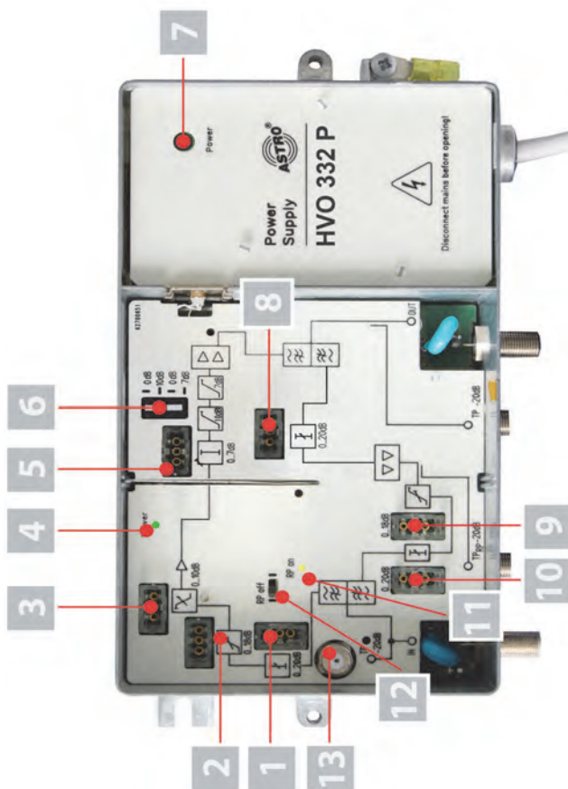
Bild 2: Verstärker HVO 332 P, Innenansicht
