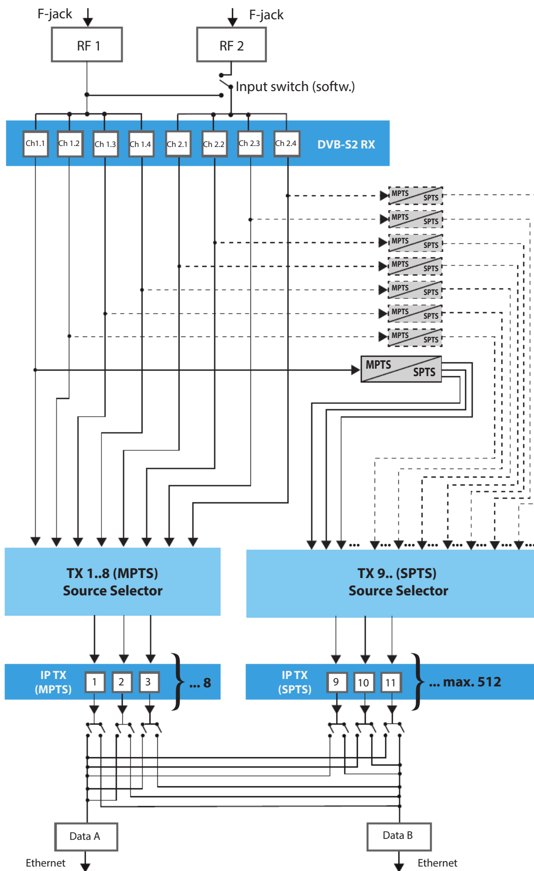
Bild 7: Signalfluss im U 168 und U 168-X
