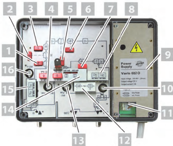
Bild 2: Verstärker VARIO 682 O, innen (VARIO 681 O ähnlich)
