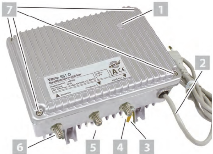
Bild 1: Verstärker VARIO 681 O (VARIO 682 O ähnlich)
